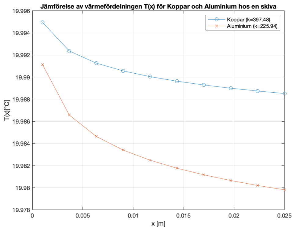
Figur 16: Graf för jämförelse av temperaturfördelningen för en skiva i aluminium respektive koppar, där x-axeln visar avståndet från centrum av skivan, där strålen träffar, och y-axeln visar temperaturen i grader Celsius.
