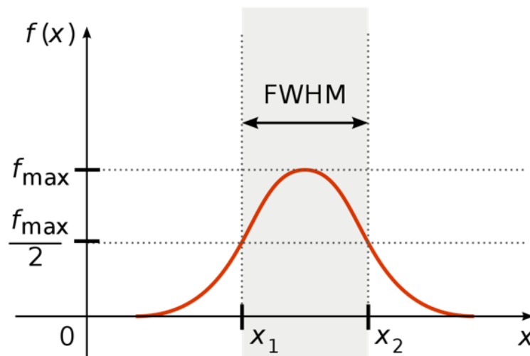
Figur 3: Beskrivande graf för definition av FWHM av Arne Nordmann återpublicerad från [7], CC BY-SA. På y-axeln är f_{\max} den maximala erhållna signalen och x_1 och x_2 är markeringar var signalen är 50% av f_{\max} . FWHM är markerat som avståndet mellan x_1 och x_2 .
