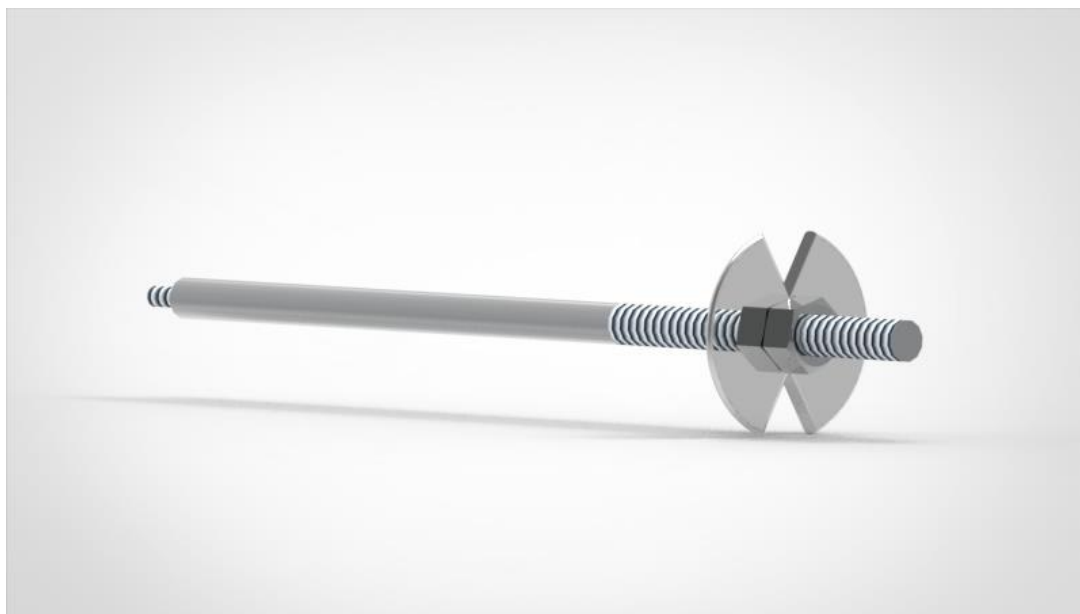
Figur 13: Rendering av roterande aluminiumskiva på drivaxeln. På baksidan är drivaxeln gängad för fäste i motorn. Framsidan av axeln är gängad för att muttrar ska hålla skivan på plats.
