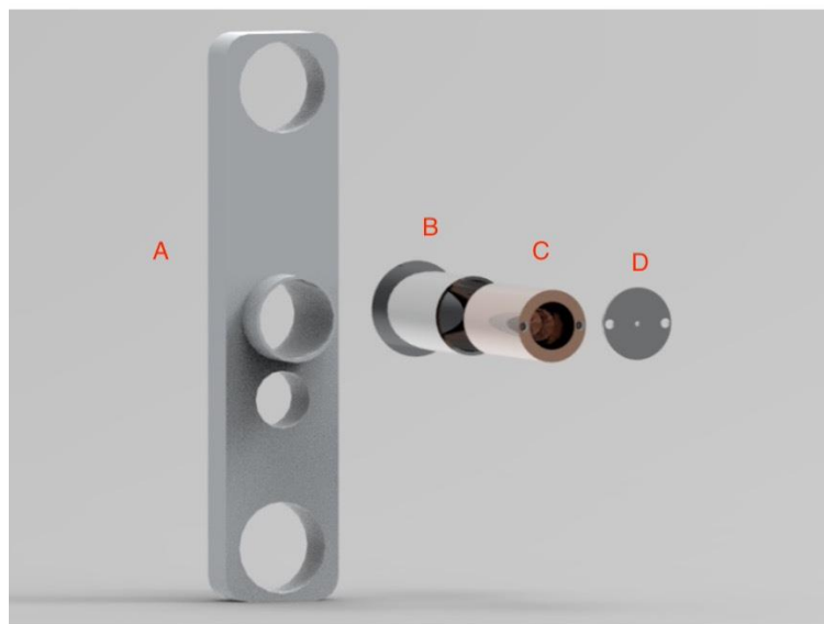
Figur 12: Rendering av Faraday-kopp bestående av stålomslutning (B) och koppar-kopp (C) placerad bredvid fästet för Faraday-koppen (A). Aperturplattan (D) är avtagen och placerad till höger om Faraday-koppen.
