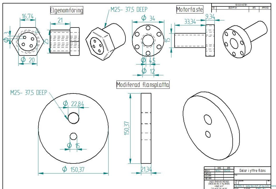
Figur 8: Ritning av elgenomföring, motorfäste samt en modifierad flänsplatta. Längst upp till vänster i bilden syns elgenomföringen, till höger syns motorfästet och nertill i figuren syns den modifierade flänsplattan.
