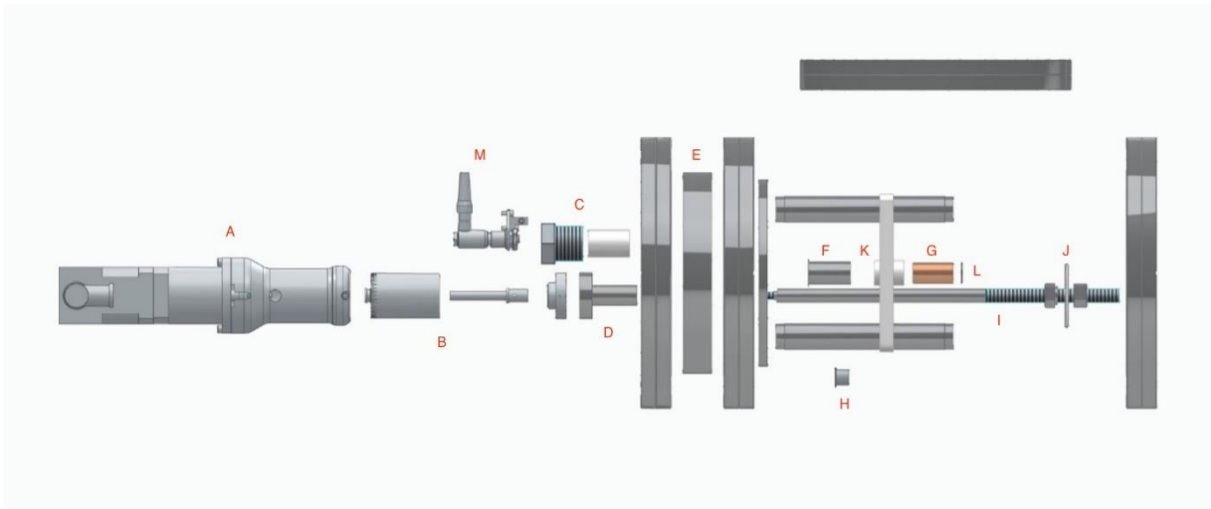
Figur 11: Uppdelad tvådimensionell vy av den kompletta uppställningen i Solid Edge. Bilden visar samtliga delar isärtagna från varandra: stegmotor (A), magnetkoppling (B), hemsensor (M), elgenomföring (C), motorfäste (D), flänsplatta (E), stålomslutning (F), glidlager (H), fäste för Faraday-kopp (K), koppar-kopp (G), aperturplatta (L), drivaxel (I) och aluminiumskiva (J).
