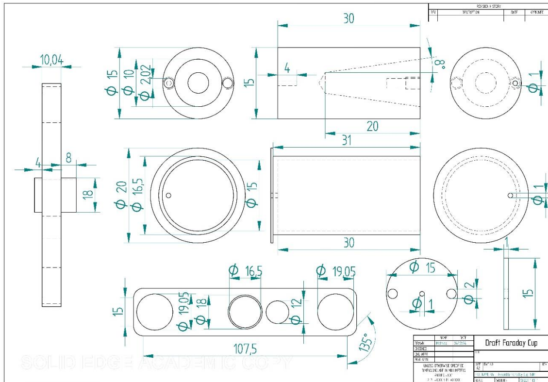
Figur 5: Figuren visar ritning av Faraday-kopp separerad i 4 delar: kopparkopp, stålomslutning, aperturplatta och fäste till Faraday-koppen. Till vänster och längst ner i bilden visas ritningen för fästet. Högst upp i figuren visas kopparkoppen framifrån, från sidan samt bakifrån. I mitten visas ritning över stålomslutningen från samma vinklar som kopparkoppen. Till sist visas aperturplattan nere i högra hörnet framifrån samt från sidan.
