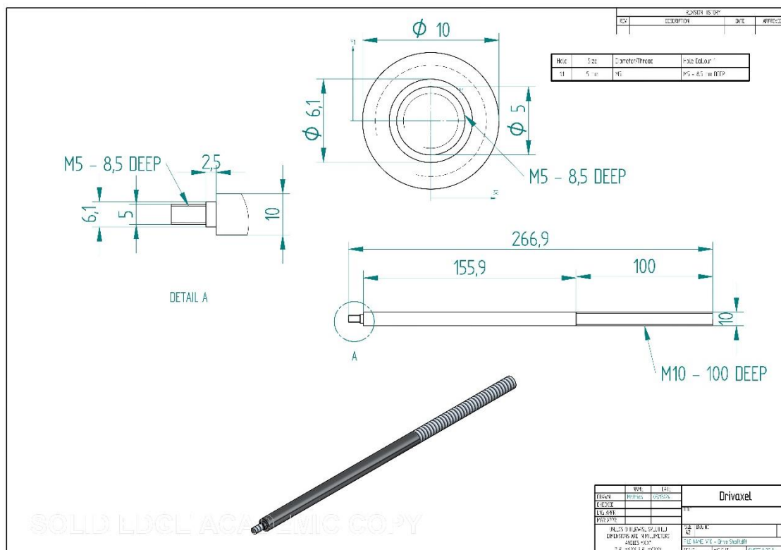
Figur 6: Ritning över drivaxeln. Ritningen innehåller en vy framifrån och en från sidan samt en detalj över området markerat som "A".
