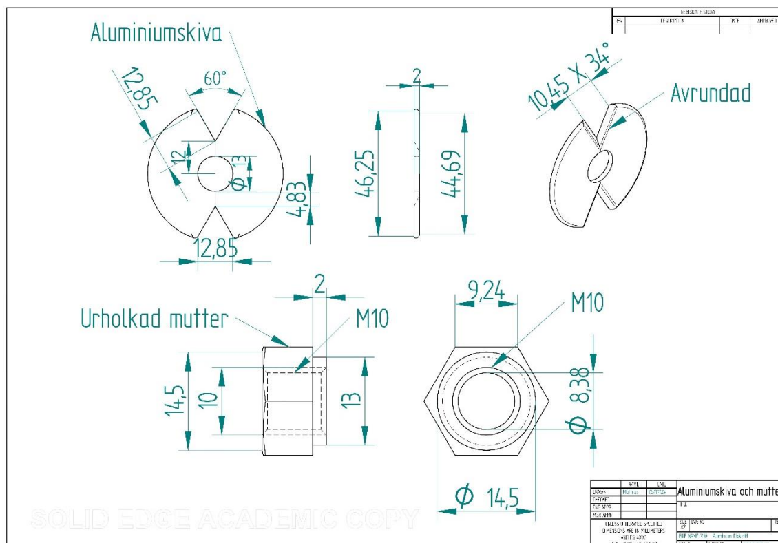
Figur 7: Ritning av aluminiumskivan samt den modifierade M10 muttern. Skivan visas ur 3 perspektiv: framifrån, från sidan samt från en sned vinkel. Muttern visas från sidan samt framifrån.
