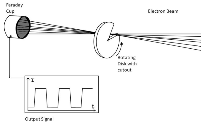
Figur 1: Förenklad experimentell uppställning återpublicerad från [4] med tillstånd av Sondur et al. Uppställningen består av en roterande skiva med cirkelsektorutskärning och en Faraday-kopp.
