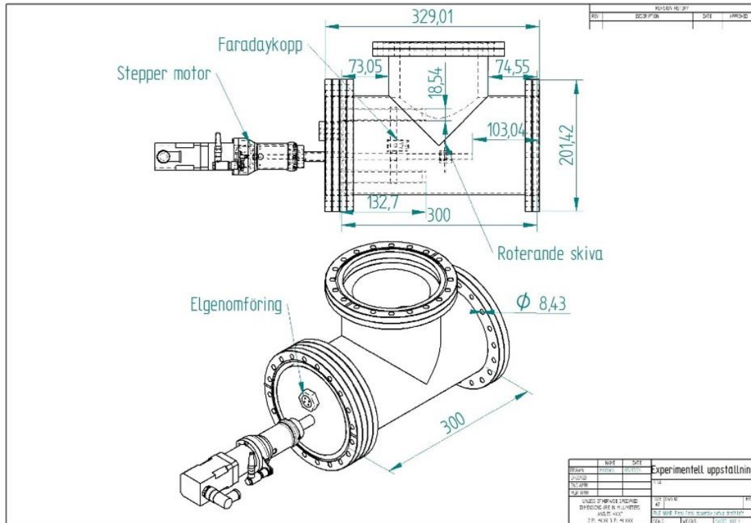
Figur 9: Visar ritning av den kompletta uppställningen. Den övre ritningen visar uppställningen från sidan medan den undre visar den snett från sidan. Huvudsakliga delar och mått är markerade i figuren.
