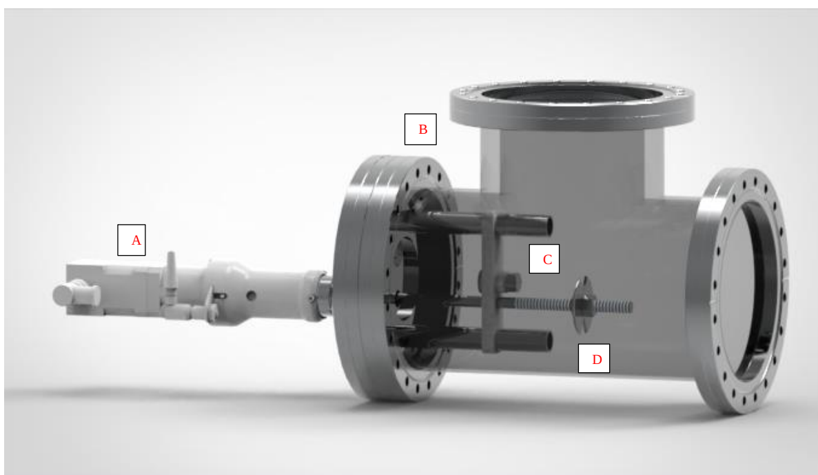
Figur 10: Rendering av den kompletta uppställningen. Uppställningen inkluderar en stegmotor (A), en vakuumcylinder (B), en Faraday-kopp (C) och en roterande aluminiumskiva på en gängad drivaxel (D).
