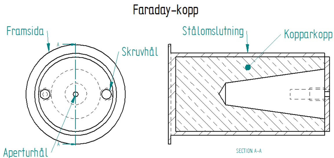
Figur 2: Ritning av Faraday-kopp designad i Solid Edge i två olika perspektiv. Figuren innehåller hela
